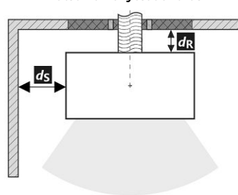
Hátsó kéménycsatlakozás
