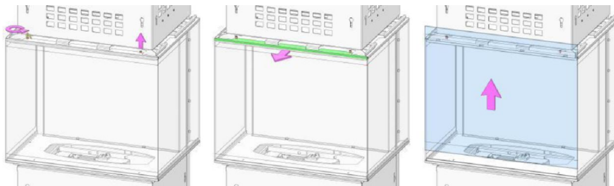
Obr. 3 Vyjmutí skla
